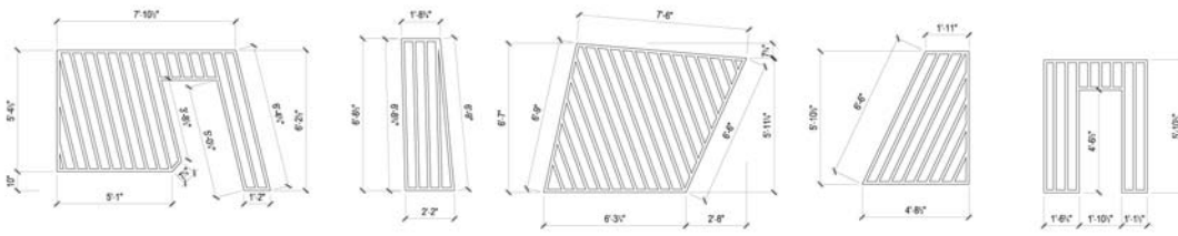
PAVILION FRAME TEMPLATES
