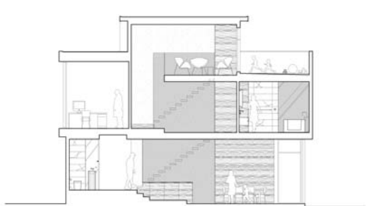
HOUSE J : SECTION
