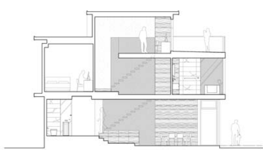
HOUSE T : SECTION
