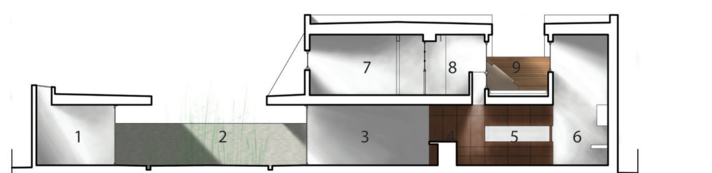
longitudinal section 0' 10'
